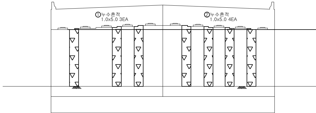
정면
