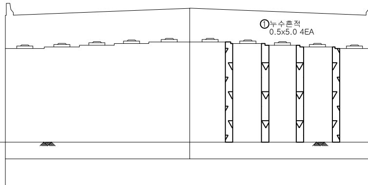
정면
